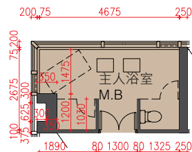
30樓的部分平面圖 PART PLAN FOR 30/F
